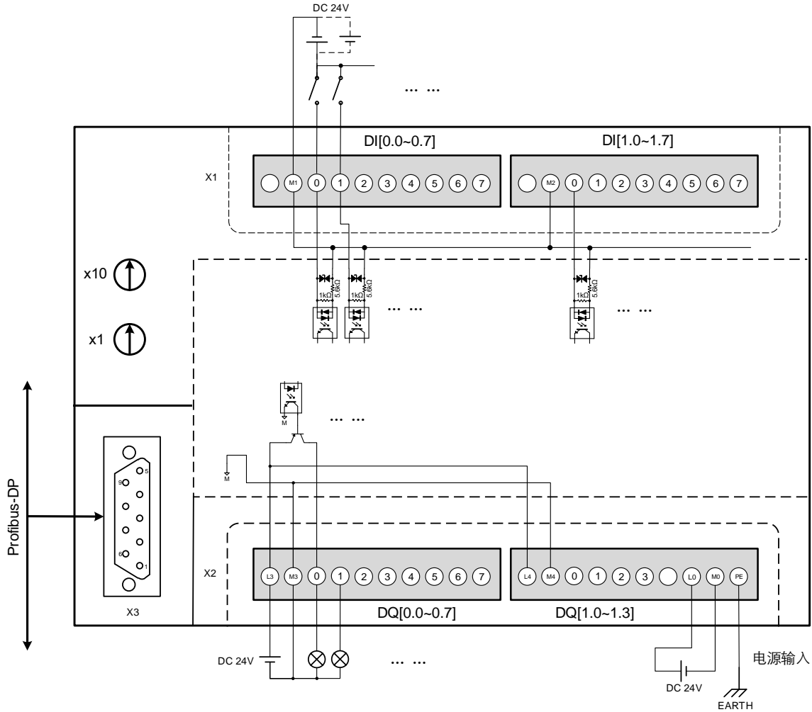
图 3 模块接线图
