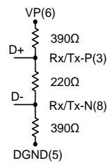
图 5 总线终端器
